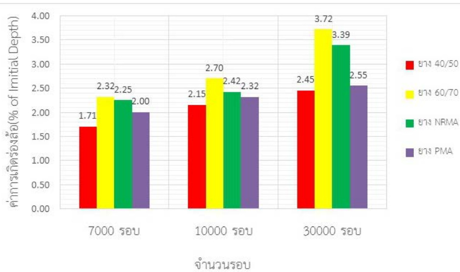
ภาพที่ 4.2 ผลการทดสอบการจำลองการเกิดร่องล้อในห้องปฏิบัติการ (กิติฤกษ์ ฉิมทับ, 2562)
