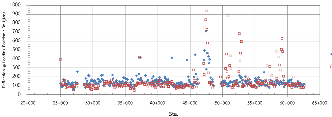
ภาพที่ 7.1 รูปแสดงค่าการยุบตัวจากการทดสอบ FWD ที่ตำแหน่ง Loading Plate ก่อนก่อสร้างและหลังการก่อสร้างประมาณ 2 ปี
