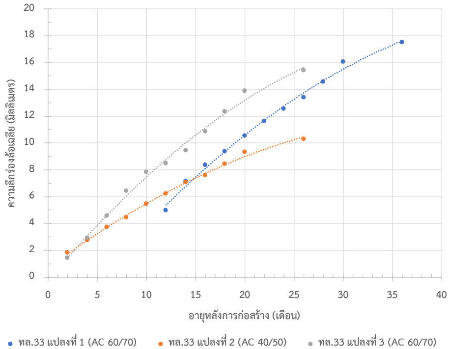
ภาพที่ 5.1 ผลการทดสอบร่องล้อ (เซซฐา สุโพธิ์, 2563)
